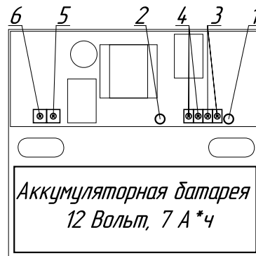
Схема подключения
